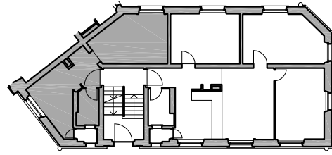
Grundriss Erdgeschoss
