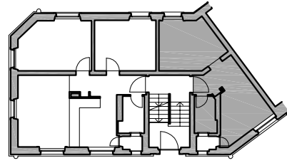
Grundriss Erdgeschoss
