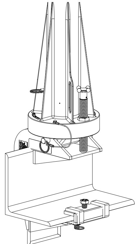
EDGE MOUNT
