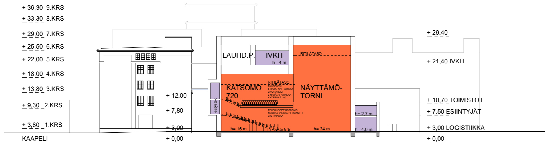
LEIKKAUS A-A
