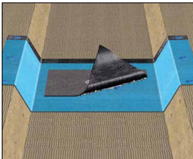
Sluket festes mekanisk, og belegget på sluket helsveises så til Base Syntanen. Det er viktig at varmen tilføres undersiden på slukbelegget og ikke direkte på syntanen.
