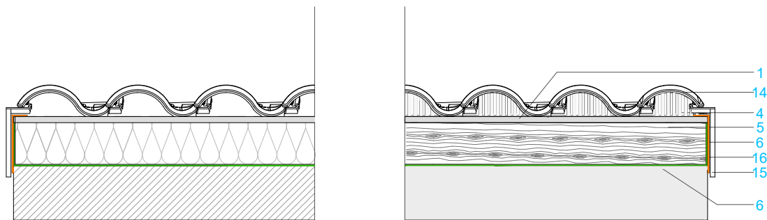
SECCIÓN 2 CUBIERTA DOS AGUAS CON TECTUM PRO
