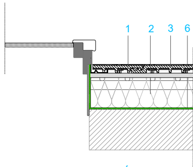
SECCIÓN 3 ENCUENTRO CON CLARABOYA
