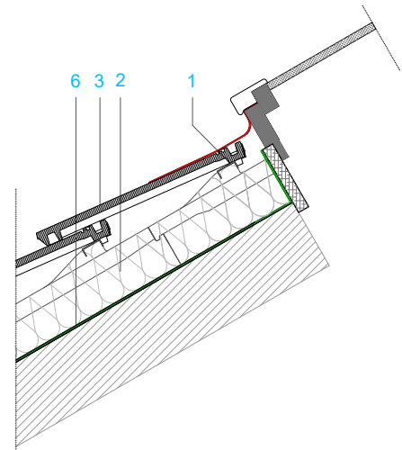
SECCIÓN 4 ENCUENTRO CON CLARABOYA
