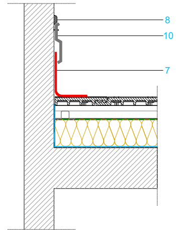
SECCIÓN 2 ENCUENTRO CON MURO LATERAL
