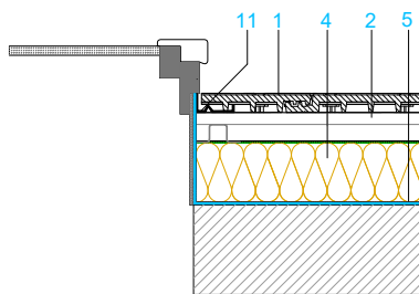
SECCIÓN 3 ENCUENTRO CON VENTANA
