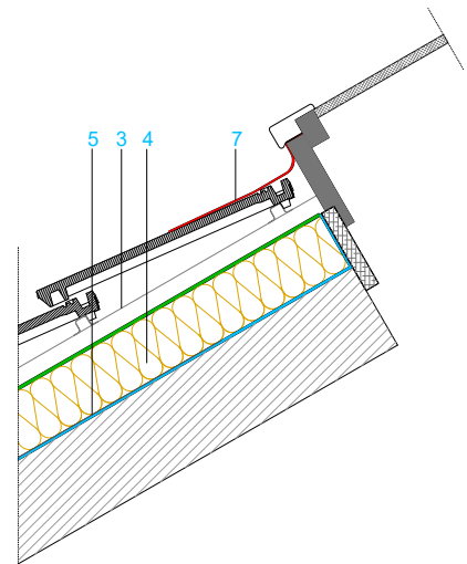
SECCIÓN 4 ENCUENTRO CON VENTANA
