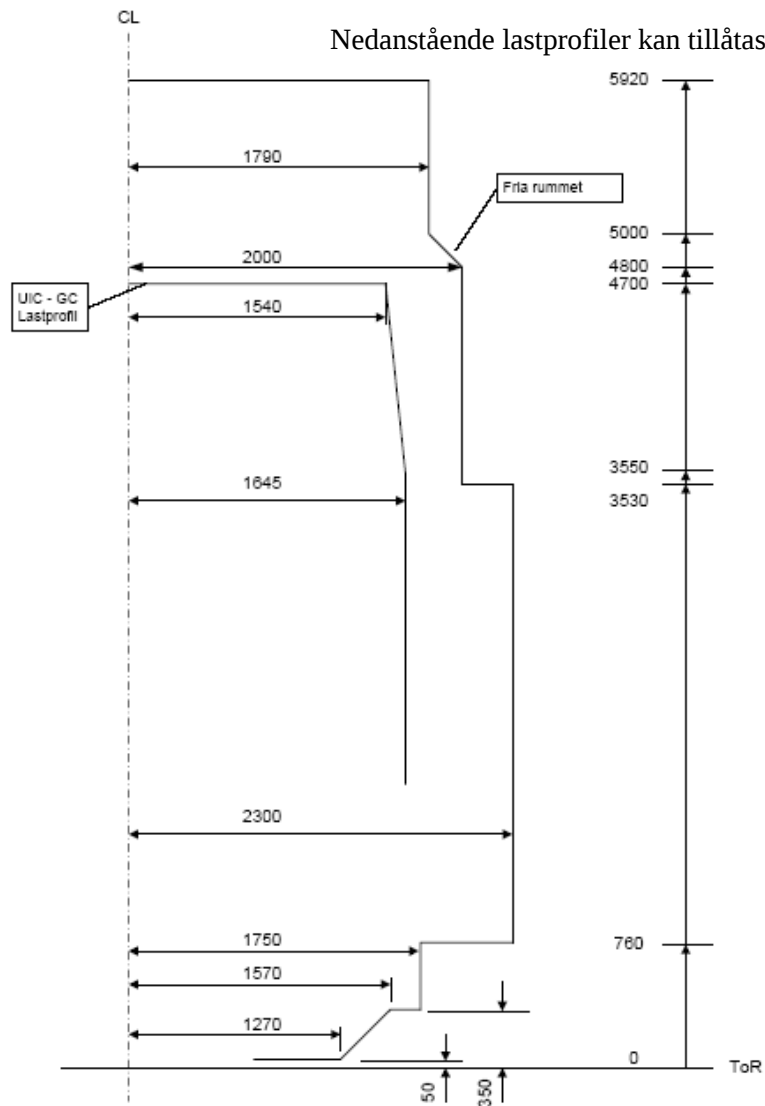
Kombiprofil P/C 450 (2,60 m x 4,83 m)
