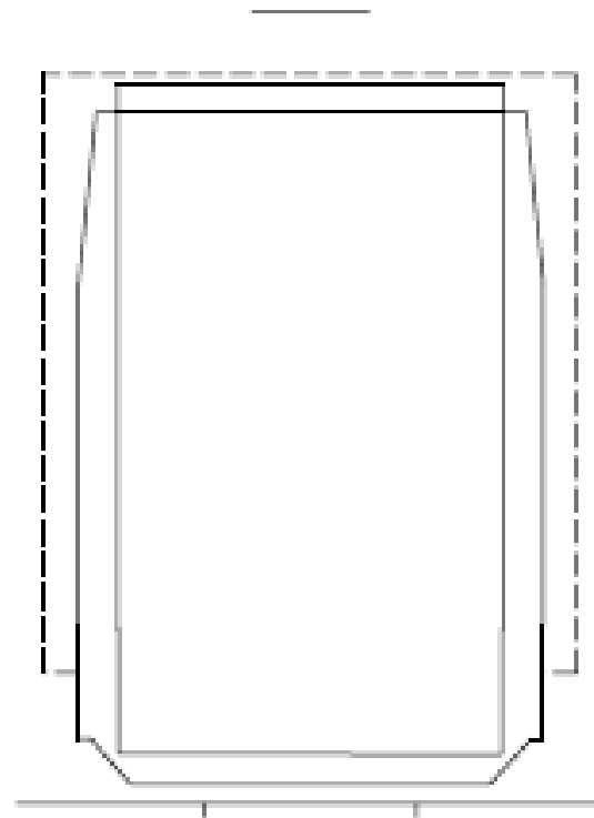
Kombiprofil P/C 450 (2,60 m x 4,83 m)
