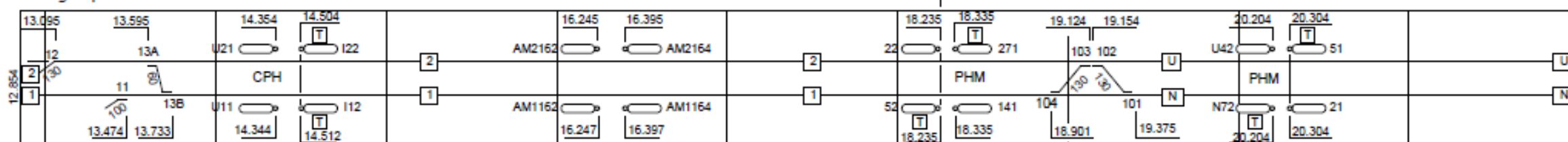
Signalplan
