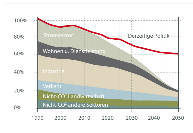
Abbildung 6: Wege zur Verringerung der THG-Emissionen in der EU um 80% (100%=1990), [EU Kommission 2011]
