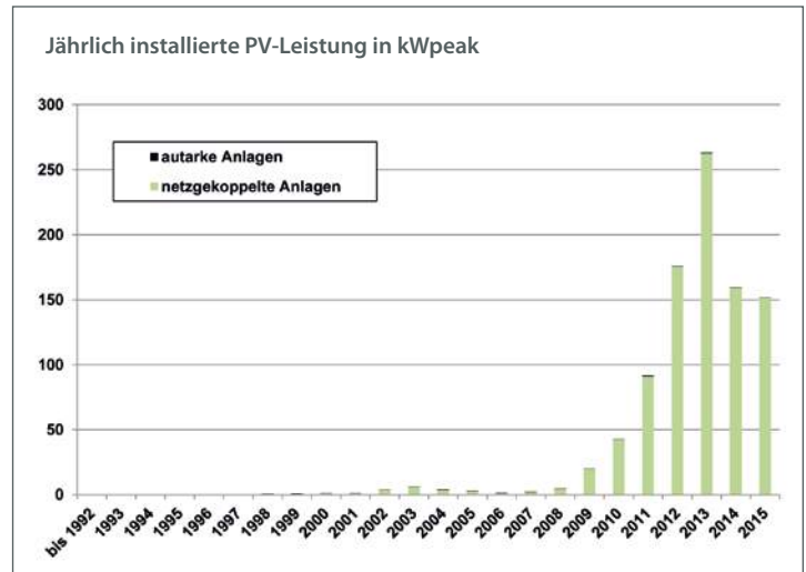
Abbildung 3: Jährlich in Österreich neu installierte PV-Leistung in kWpeak der Jahre 1992 bis 2015. Quellen: bis 2006: Faninger (2007); ab 2007: Erhebung Technikum Wien, [Biermayr et al. 2015] Anmerkung: Im Jahr 2013 erhöhte eine zusätzliche Förderung, die auf dem Abbau einer Warteliste beruhte, die Installationsraten.
