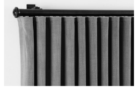
RIPPLEFOLD
