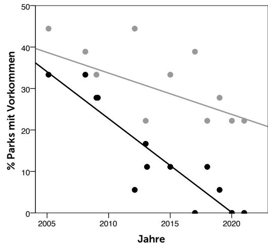
Abb. 4: Anteil an Stadtparks mit Haussperlingsvorkommen im Zeitraum 2005-2021, getrennt dargestellt für Parks, die in eine unterschiedlich stark versiegelte urbane Matrix eingebettet sind (graue Linie: Versiegelungsgrad > 75 %, schwarze Linie: Versiegelungsgrad \leq 75 %).
