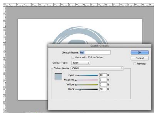
Afbeelding 2 - Spotkleur aanmaken
