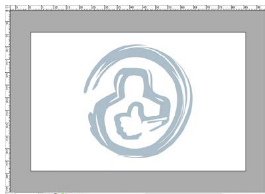
Afbeelding 3 - Weergave spotkleur
