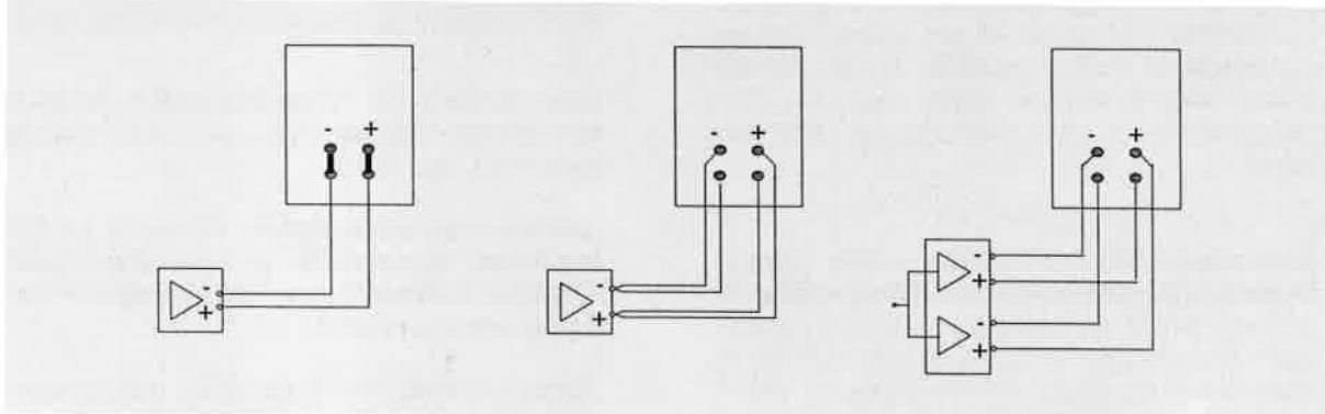
Kuva 1. Normaali johdotus
