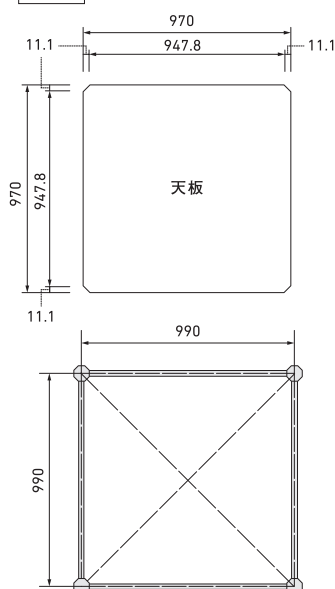
天面図
