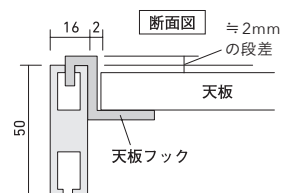
断面図
