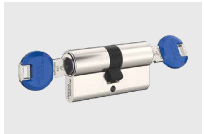
Beidseitig-sperrbarer-Zylinder (Sonderfunktion)
