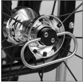
MG 28 Tetraentriegelung
