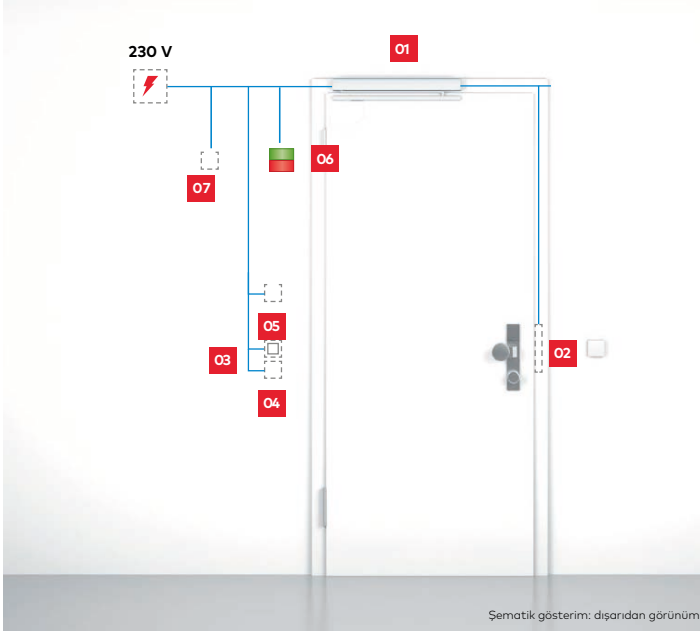
Otomatik pivot kanat açma mekanizması ED, 100/250
