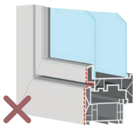
flächenbündig
