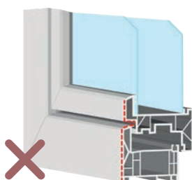
Fenêtres affleurantes
