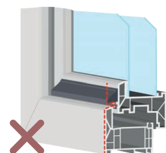
flächenversetztes Fenster mit Wetterschenkel
