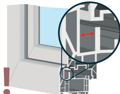
Mitteldichtung: Abstand mind. 10 mm
