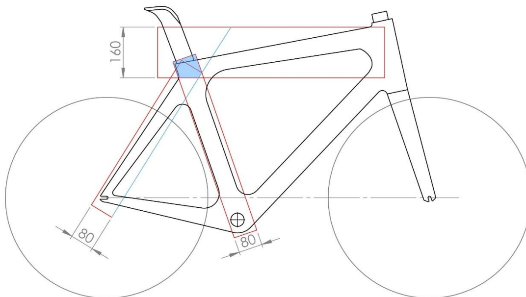
Figure 29 : Illustration de la règle sur l'inclinaison des haubans
