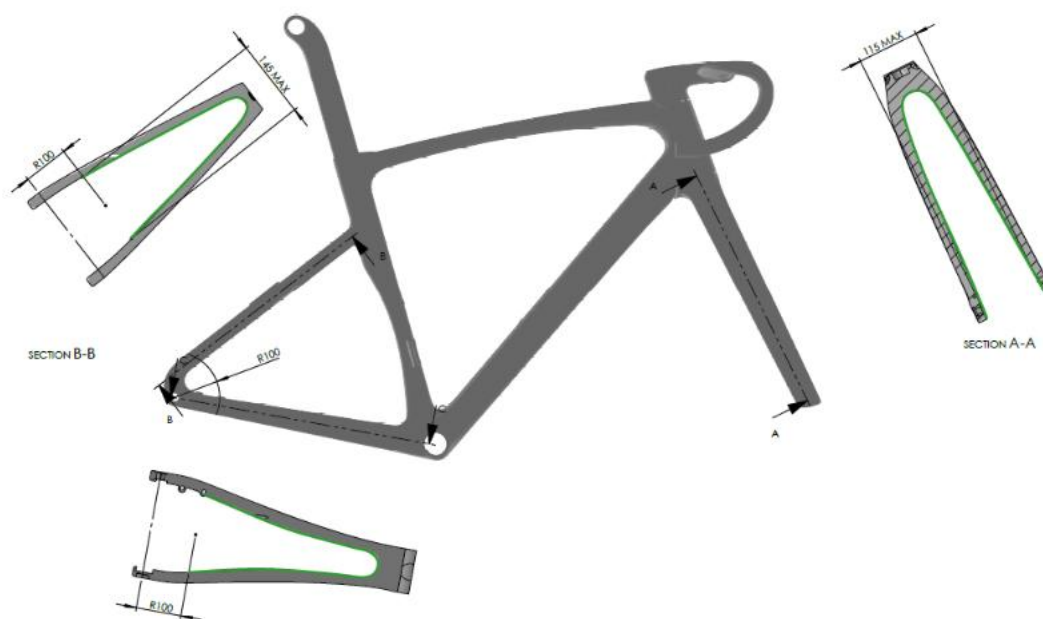
Figure 9: Route et cyclo-cross – Illustration des distances entre les fourreaux de la fourche et entre les haubans arrières.
