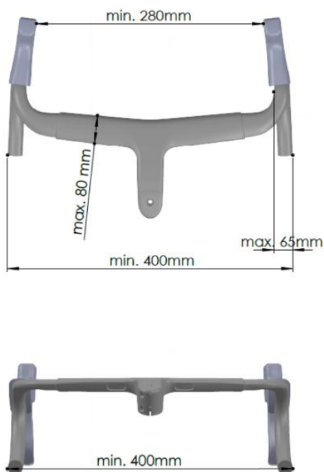
Figure 37 Route et Cyclo-Cross, Illustration d'un guidon qui doit se conformer avec une largeur minimale de 400mm.
