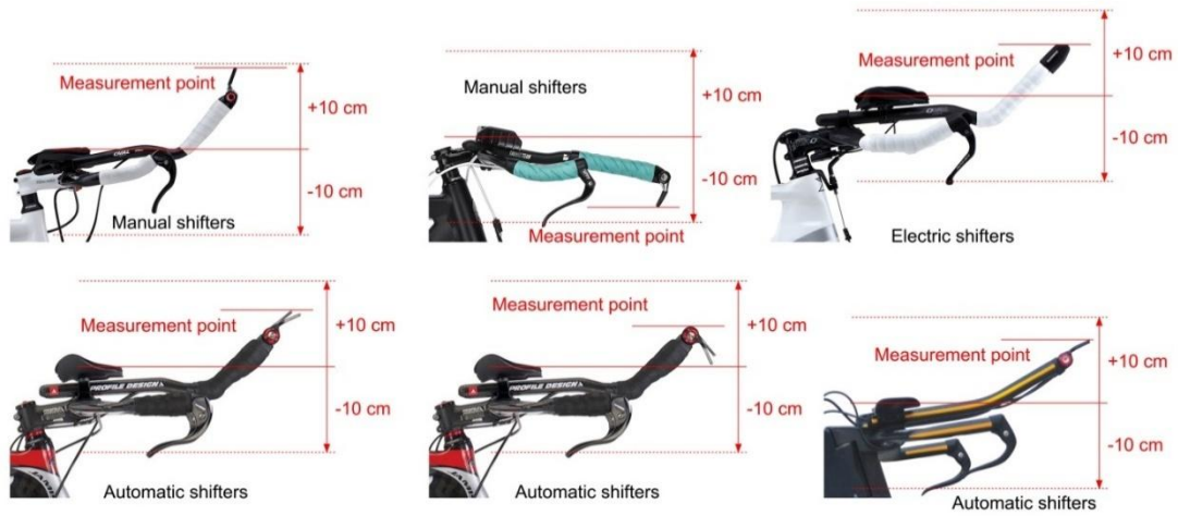
Figure 53 : Points de mesure pour les limites verticales de l'extension fixe additionnelle du guidon de contre-la-montre avec tous ses accessoires
