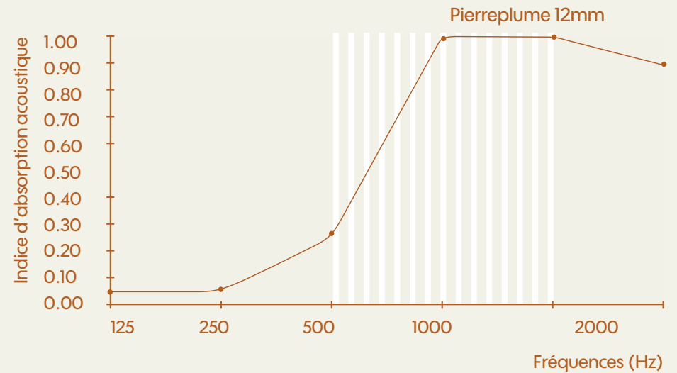
Courbe du coefficient d'absorption acoustique pratique conformément à la norme NF EN ISO 354
