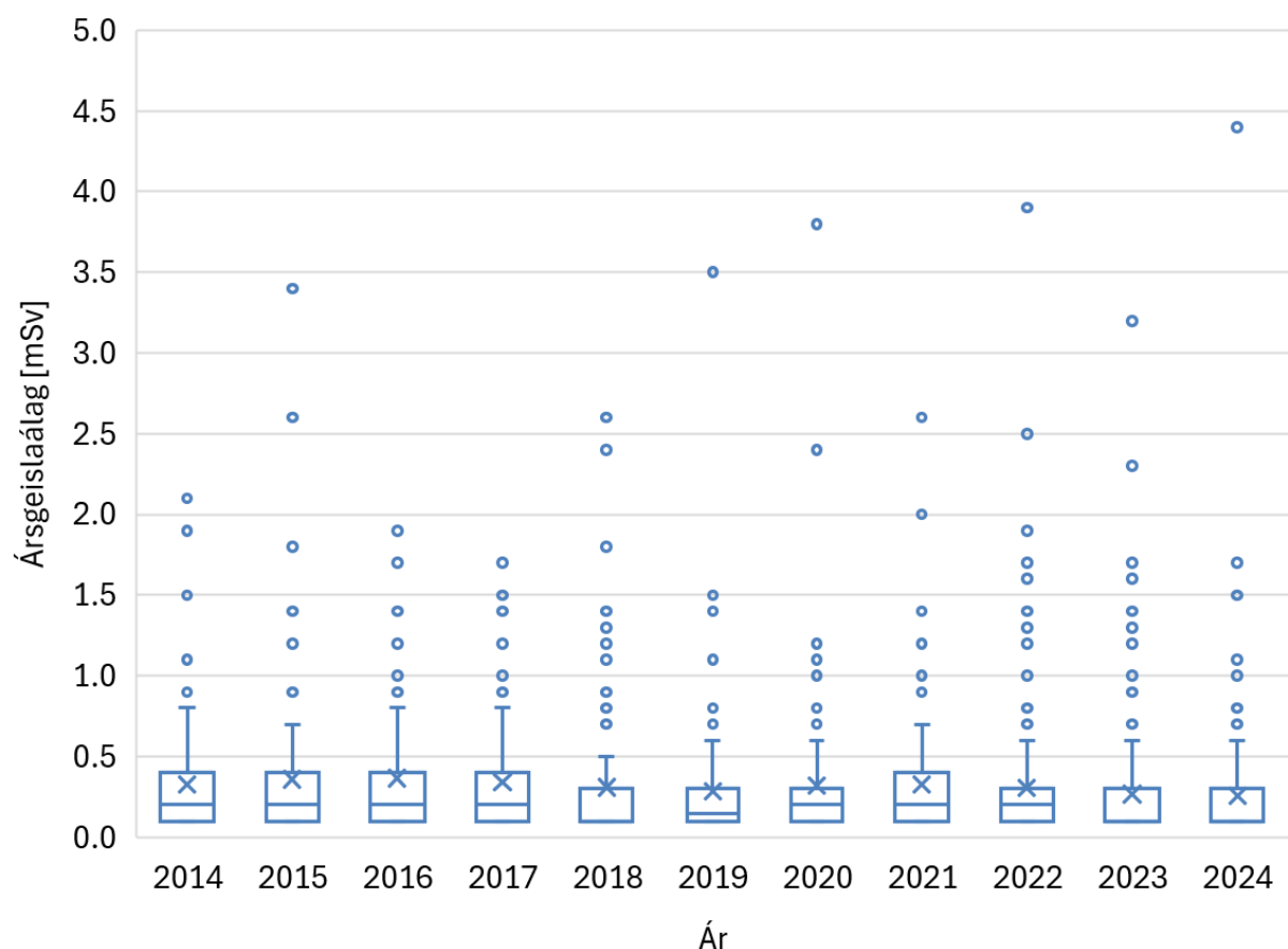
Mynd 1: Dreifing ársgeislaálags fyrir starfsmenn með mælanlegt geislaálag ( E > 0 ), fyrir árin 2014 – 2024. Bláir kassar sýna fjórðungaspönn fyrir hvert ár og línur innan þeirra sýna miðgildi geislaálags (árin 2018, 2023 og 2024 var miðgildi geislaálags jafnt neðra fjórðungsmarki). Meðalársgeislaálag er merkt með X-i. Bláu línurnar fyrir utan kassana ná að hæsta og lægsta gildi nema ef um er að ræða útlaga (bláir hringir), þ.e.a.s. gildi sem eru lengra frá lægra eða efra fjórðungsmarki en sem nemur einni og hálfri fjórðungaspönn. (Distribution of annual effective dose for the years 2014 – 2024. Boxes show the interquartile range and horizontal lines within boxes show the median annual effective dose (median annual effective dose for the years 2018, 2023 and 2024 was equal to the 25th quartile). Average annual effective dose is shown with a cross. Whiskers show the maximum and minimum values, except for outliers shown as blue circles (outliers defined as values lying more than 1,5 times the interquartile range away from either quartile). Data shown only for monitored workers with annual effective dose E > 0 .)
