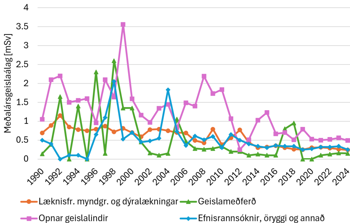
Mynd 7: Meðaltal ársgeislaálags E flokkað eftir starfssviðum fyrir árin 1990 – 2024, fyrir starfsmenn með ársgeislaálag E > 0 . (Average annual effective dose E categorized by occupational field for the years 1990 – 2024. Data shown only for monitored workers with effective dose E > 0 .)
