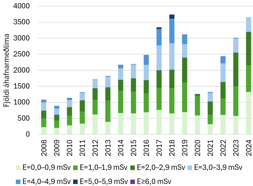
Mynd 9: Ársgeislaálag flugáhafnarmeðlima flokkað eftir stærðarflokkum geislaálags fyrir árin 2008 – 2024. (Flight crew annual effective dose E categorized by annual effective dose for the years 2008 – 2024).
