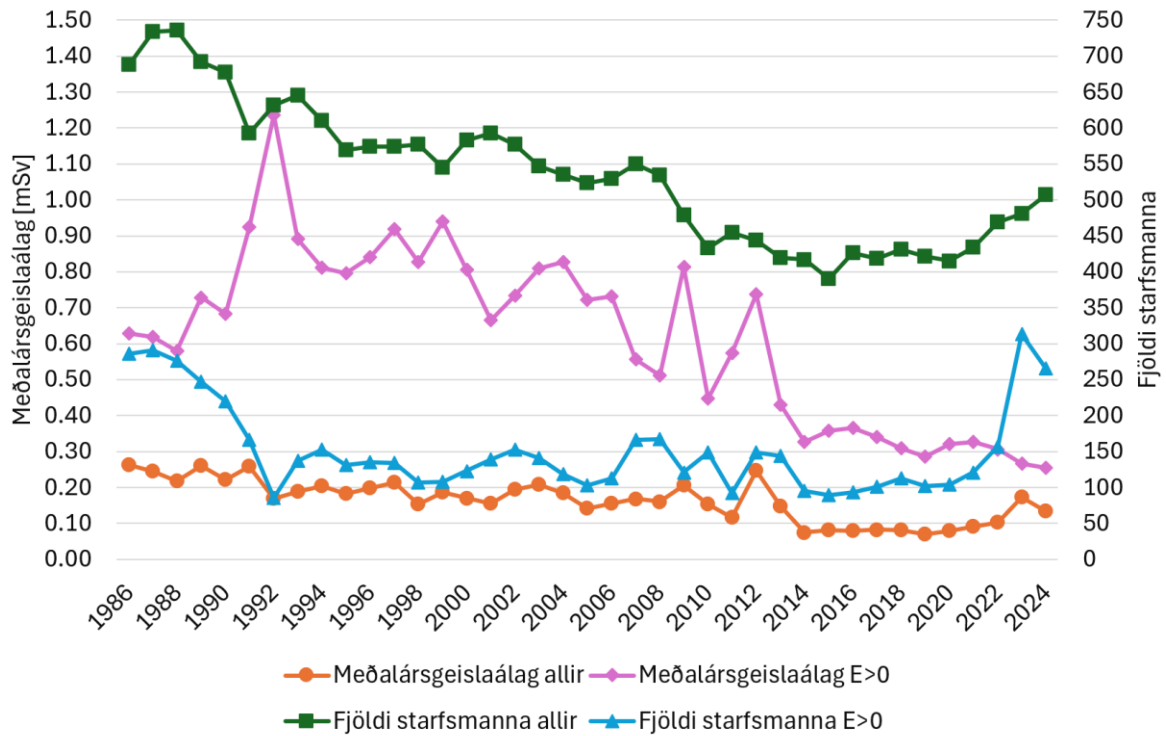
Mynd 2: Meðaltal ársgeislaálags E og fjöldi starfsmanna sem báru einstaklingsmæla árin 1986 – 2024. Gögn sýnd fyrir alla starfsmenn sem báru einstaklingsmæla og fyrir starfsmenn með mælanlegt ársgeislaálag E>0. (Average annual effective dose E and no. of workers who carried personal dosimeters for the years 1986 – 2024. Data shown for all monitored workers and for workers with annual effective dose E>0.)
