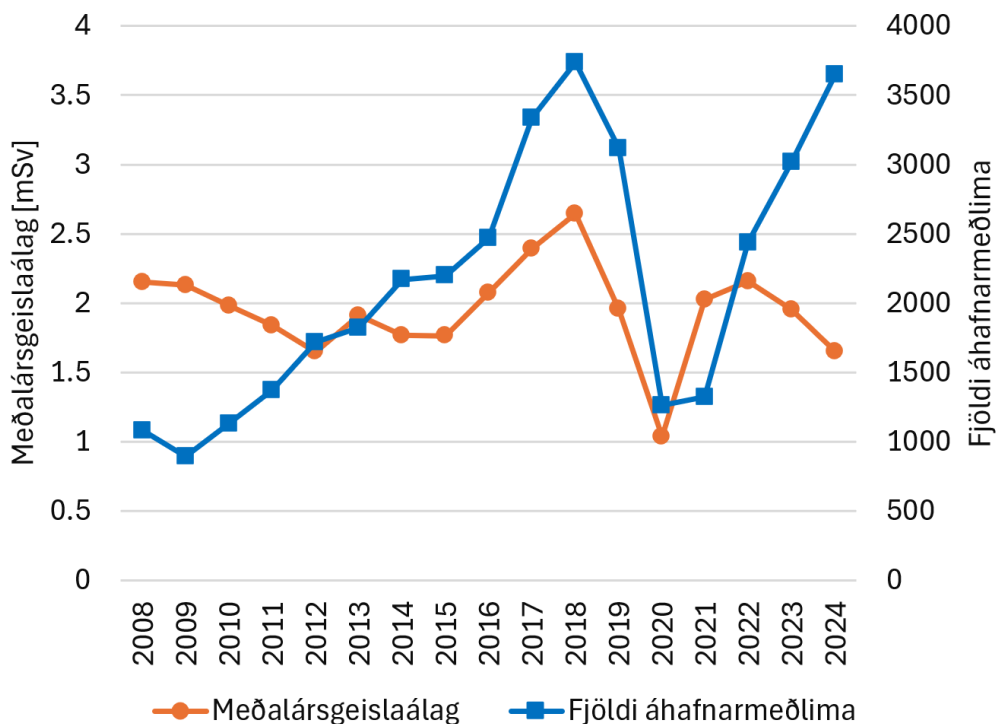
Mynd 8: Meðalársgeislaálag flugáhafnarmeðlima og fjöldi áhafnarmeðlima með áætlað ársgeislaálag, fyrir árin 2008 – 2024. (Average annual effective dose of flight crew and number of flight crew with reported annual effective dose, for the years 2008 – 2024.)
