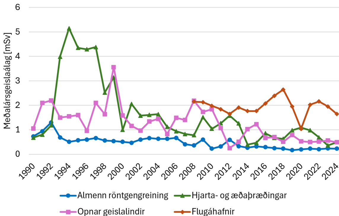
Mynd 10: Meðalársgeislaálag nokkurra starfssviða, fyrir starfsmenn með ársgeislaálag E > 0 , og flugáhafna fyrir árin 1990 – 2024. (Annual effective dose E categorized by occupational field for the years 1990 – 2024. Data shown for flight crews and monitored workers with effective dose E > 0 .)
