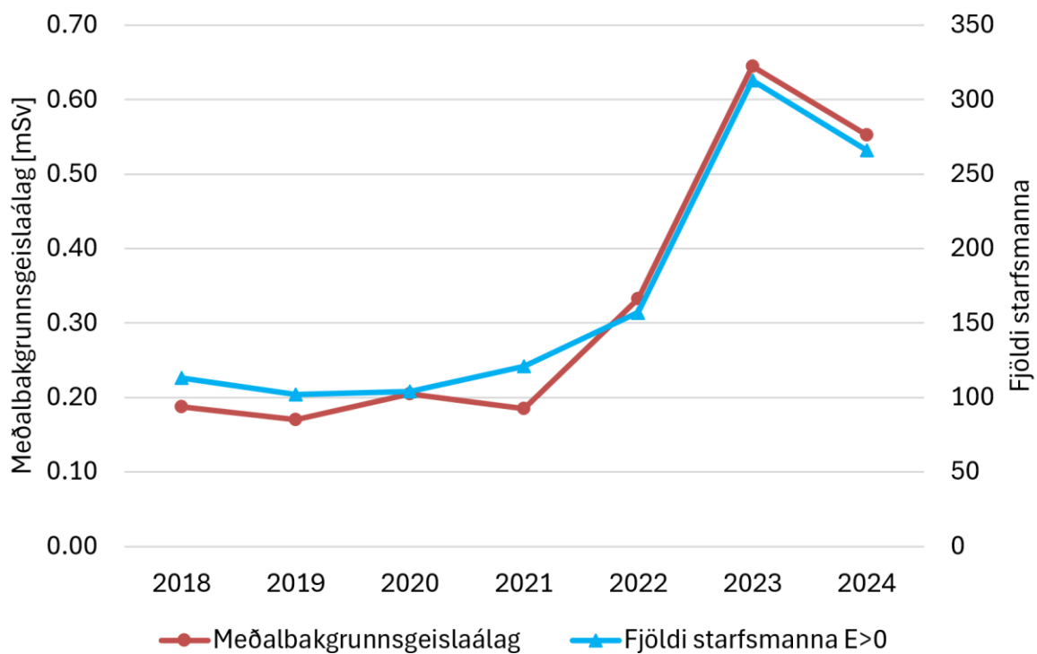
Mynd 6: Meðalbakgrunnsgeislaálag mælt með flutningsgeisla-mælum sem fylgja TLD sendingum til og frá Íslandi fyrir árin 2018 – 2024. Einnig sýndur fjöldi starfsmanna sem báru einstaklingsmæla með mælanlegt geislaálag E > 0 mSv á sama tímabili. (Average background dose measured using transport dosimeters that accompany TLD deliveries to and from Iceland for the years 2018 – 2024. Also shown is the no. of monitored workers with effective dose E > 0 during the years 2018 – 2024.)
