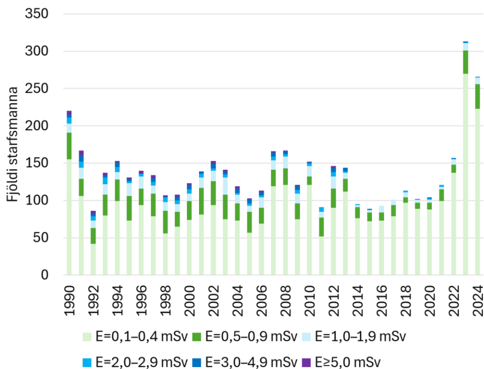
Mynd 4: Ársgeislaálag E flokkað eftir stærðarflokkum geislaálags fyrir árin 1990 – 2024, fyrir starfsmenn með ársgeislaálag E > 0 . (Annual effective dose E categorized by annual effective dose for the years 1990 – 2024. Data shown only for monitored workers with annual effective dose E > 0 .)
