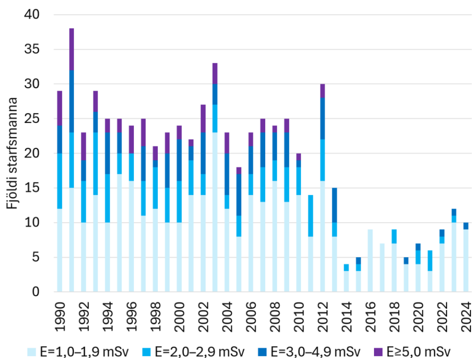
Mynd 5: Ársgeislaálag E flokkað eftir stærðarflokkum geislaálags fyrir árin 1990 – 2024, fyrir starfsmenn með ársgeislaálag E \geq 1 mSv. (Annual effective dose E categorized by annual effective dose for the years 1990 – 2024. Data shown only for monitored workers with effective dose E \geq 1 mSv.)
