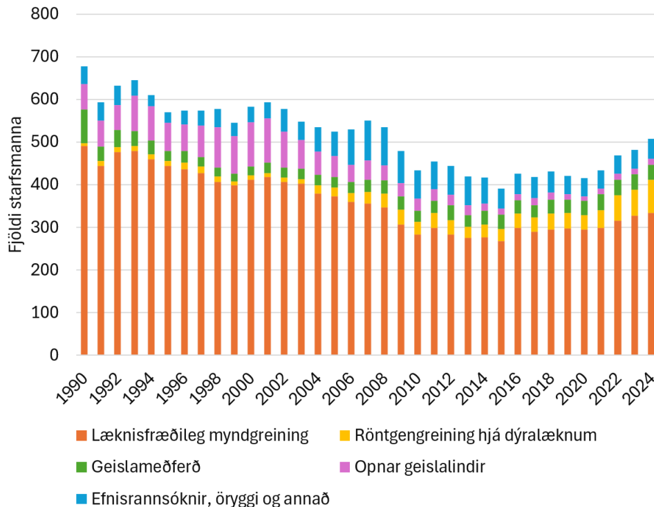
Mynd 3: Fjöldi starfsmanna sem báru einstaklingsmæla á árunum 1990 – 2024, flokkað eftir yfirflokkum starfssviða (gögn fyrir læknisfræðilega myndgreiningu og röntgengreiningu hjá dýralæknum sýnd sér). (Number of all monitored workers during the years 1990 – 2024, categorized by occupational field.)
