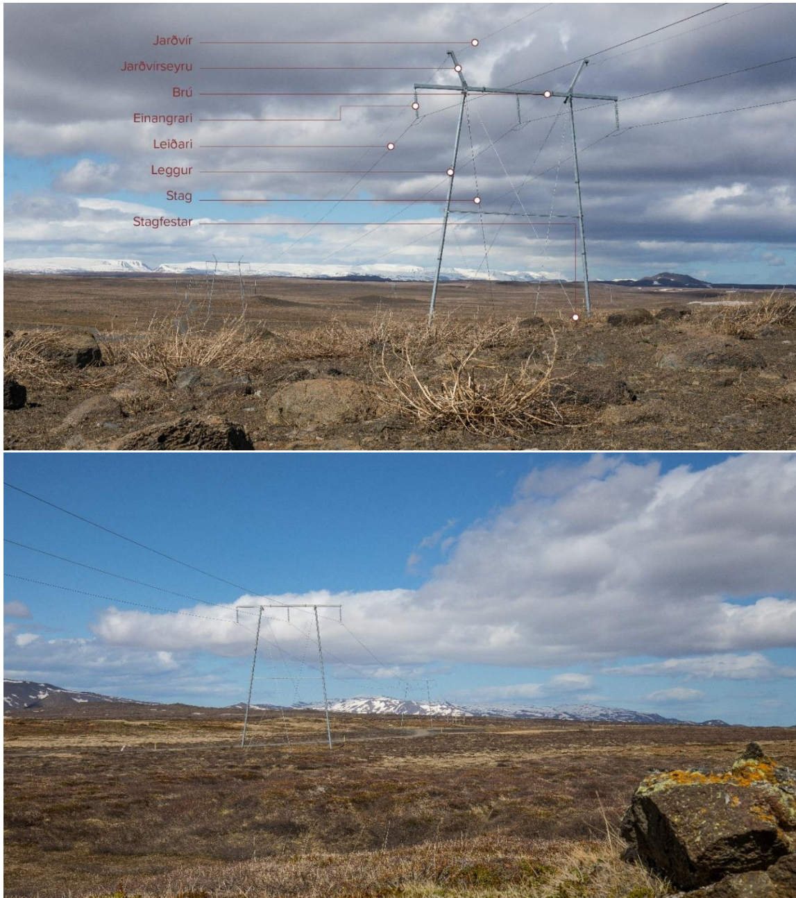
Mynd 3.1 Mastursgerð sem stefnt er að því að nota í Blöndulínu 3. Efri mynd sýnir mastur með jarðvirseyrum og neðri mynd mastur án jarðvirseyrna eins og flest möstrin í línunni verða.
