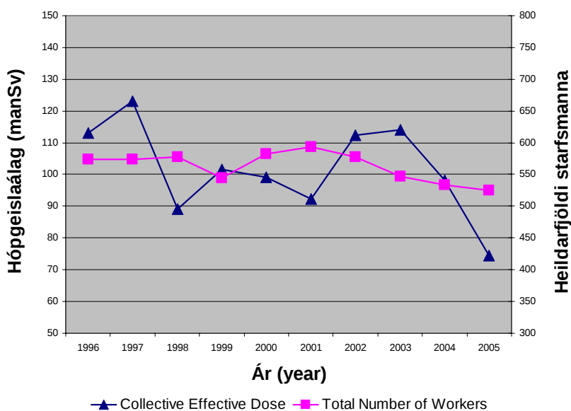
Mynd 3. Þróun hópgeislaálags og fjöldi starfsmanna með mælifilmur á árunum 1996-2005. Collective Effective Dose and the total number of workers monitored in 1996 - 2005
