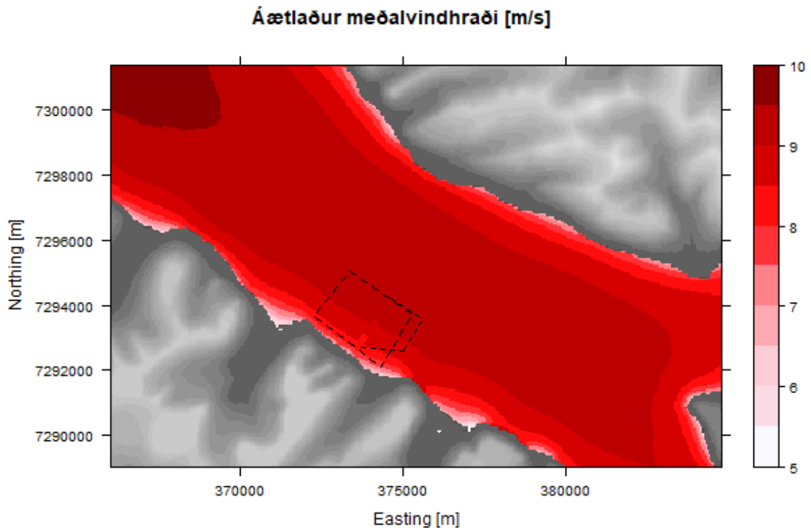
MYND 24 Yfirlitsmynd sem sýnir meðaltal 10 mín. meðalvinds í m/s skv. líkanreikningum sem byggja á mælingum frá Hálfðáni. Fiskeldissvæðið við Hringsdal er merkt inn með brotalínu. Hnitasetning er skv. UTM belti 27.
