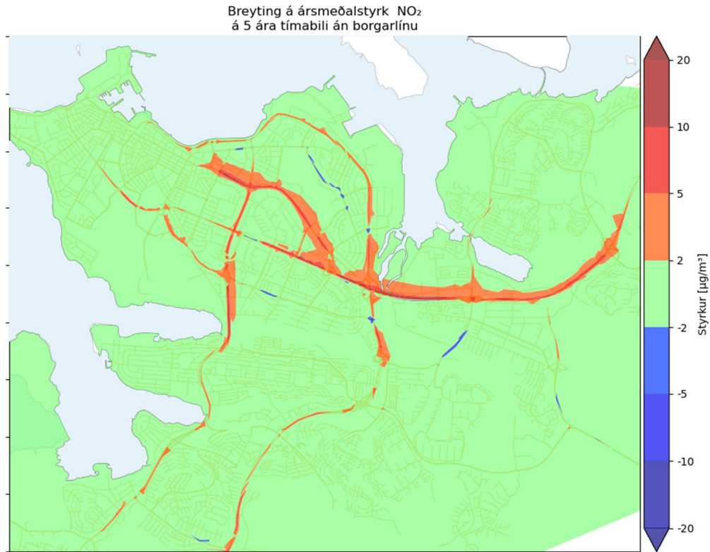
Mynd 25. Mismunur á framtíðartilviki án Borgarlínu og grunntilviki, meðalstyrkur \text{NO}_2 .
