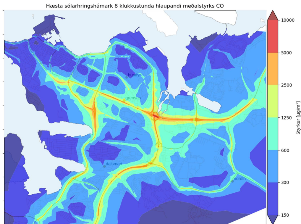
Mynd 32. Grunnástand, hæsta sólarhringsgildi 8 klukkustunda hlaupandi meðaltals CO. Umhverfismörk eru 10000 \mu\text{g}/\text{m}^3 .
