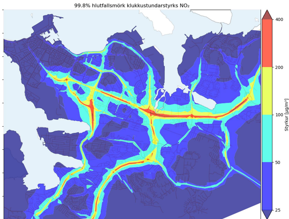
Mynd 30. Framtíðartilvik án Borgarlínu, 99,8% hlutfallsmörk klukkustundarstyrks NO 2 . Umhverfismörk eru 200 µg/m³.
