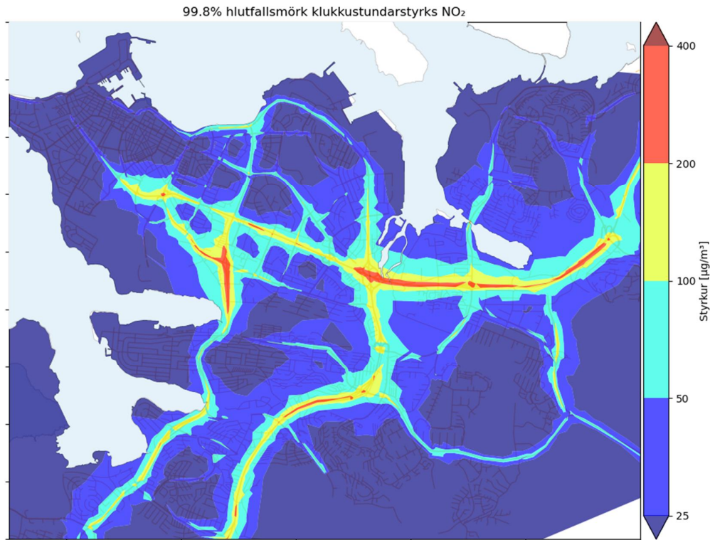
Mynd 29. Grunntilvik, 99,8% hlutfallsmörk klukkustundarstyrks NO 2 . Umhverfismörk eru 200 µg/m³.
