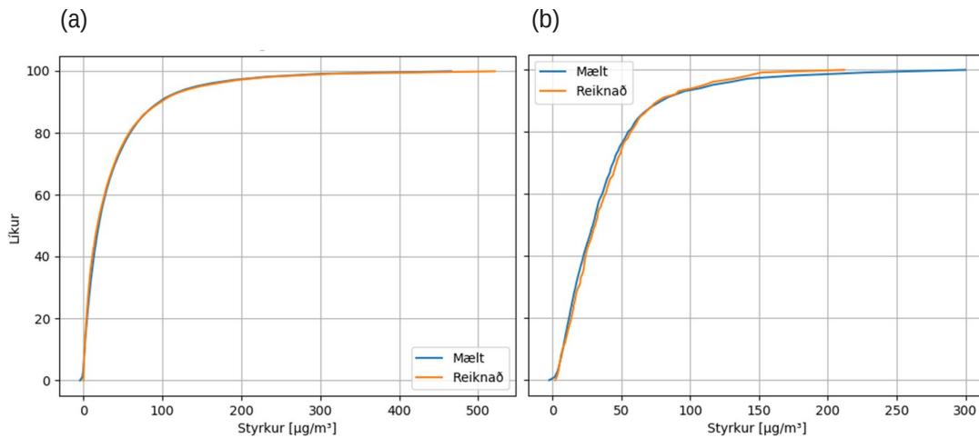
Mynd 1. Líkindadreifing klukkustundar meðalstyrks NO x (a) og sólarhringsmeðalstyrks (b), mælt 2010-2019 og reiknað 2010-2011 á Grensásvegi.
