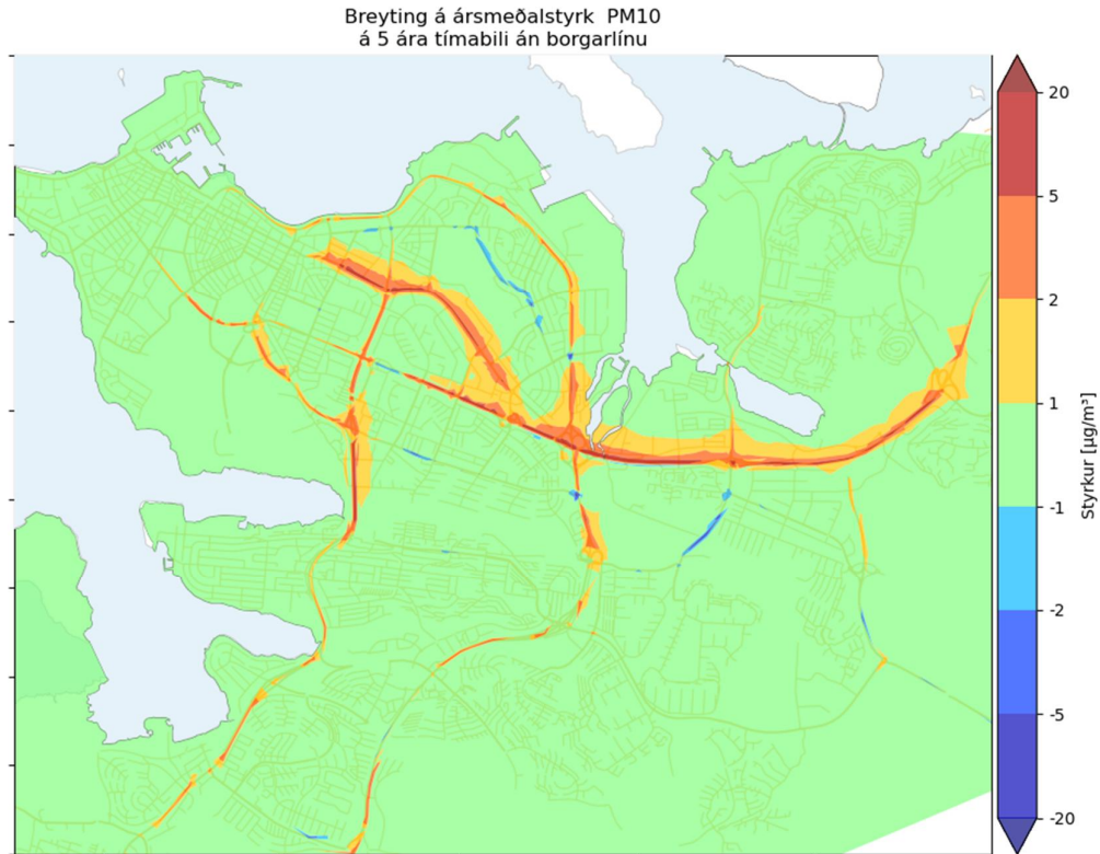
Mynd 37. Mismunur á framtíðartilviki án Borgarlínu og grunntilviki, meðalstyrkur PM 10 .
