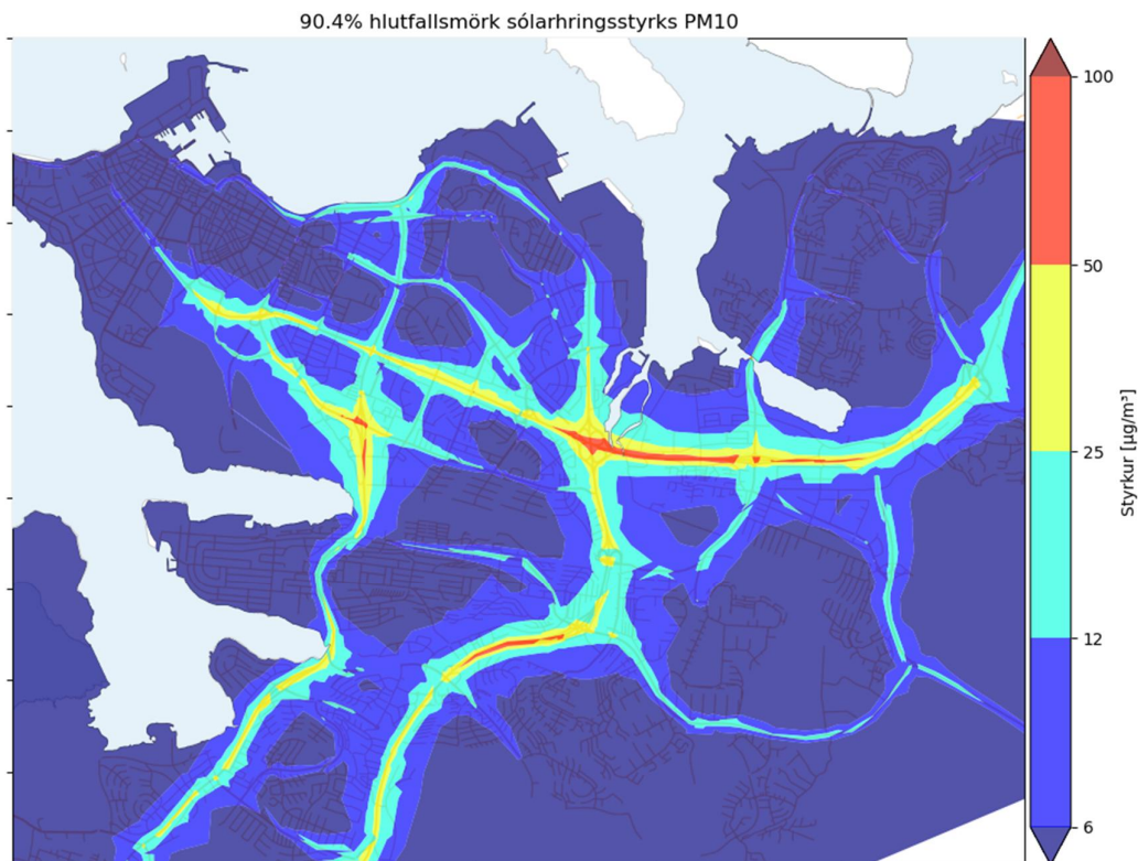
Mynd 38. Grunntilvik, 90,4 %hlutfallsmörk sólarhringsstyrks PM 10 . Umhverfismörk eru 50 \mu\text{g}/\text{m}^3 .
