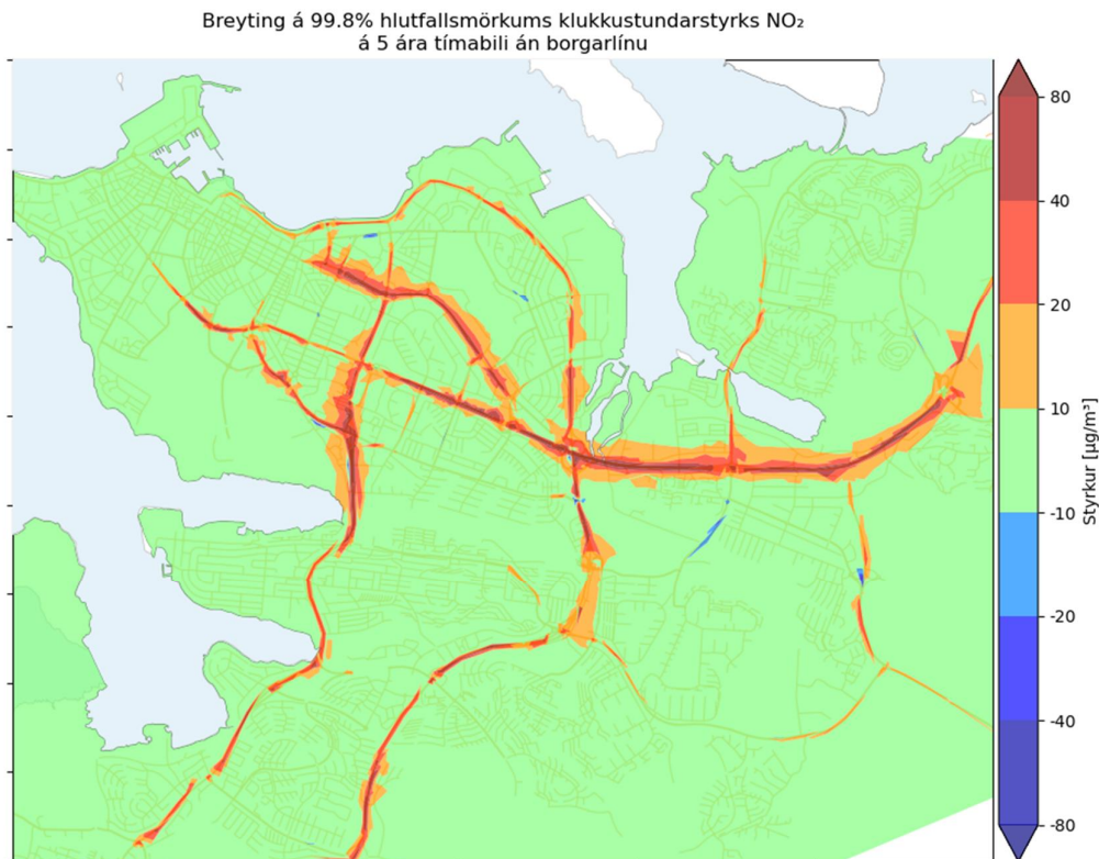
Mynd 31. Mismunur á framtíðartilviki án Borgarlínu og grunntilviki, 98,1% hlutfallsmörk sólarhringsstyrks \text{NO}_2 .
