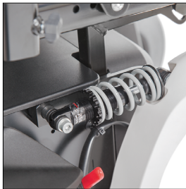
EF001 Lenradschwinge, gefedert
