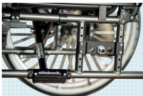
► Adapter koła tylnego flex
