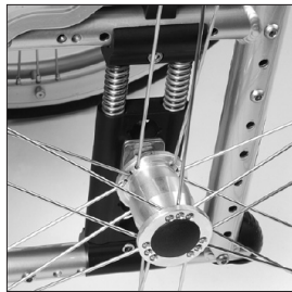
MG 97-99 Schock demper
