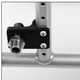
Fixation de la roue arrière
