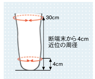
6Y95 の採寸例
