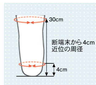
6Y95 の採寸例
