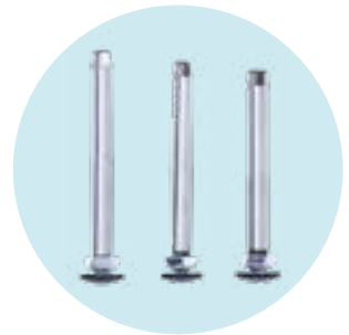
MZ81 to MZ83 Axe enfichable adaptateur avec verrouillage rapide, raccord 12 mm, roue motrice 12,7 mm
