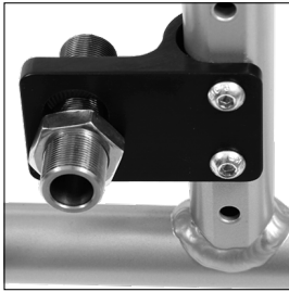
Antriebsradanbindung
