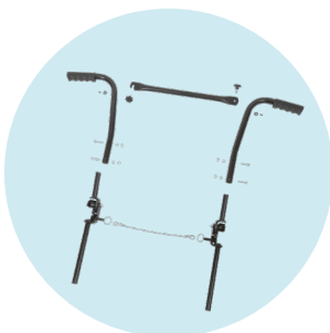
MD10 Rückenwinkelverstellung 30°
