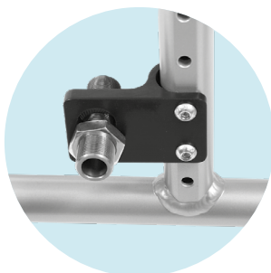
Antriebsrad-Adapter
