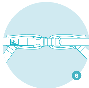
Gepolsterter 4-Punkt-Gurt
