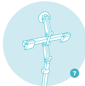
Kopfstützenhalterung mit Gurthalterung
