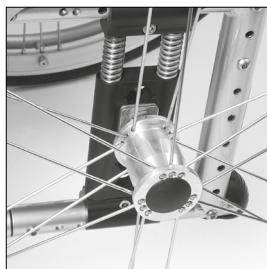
MG 97 – 99 Amortisseurs arrière Shock absorber
