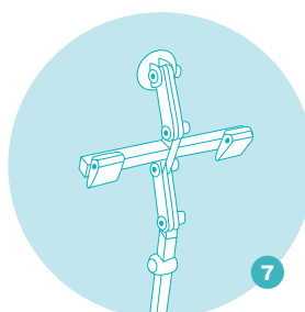
Support d'appuie-tête avec support de ceinture
