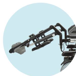
EB003 Repose-pieds relevable électr., avec compensation de lon- gueur et contrôlable séparément
