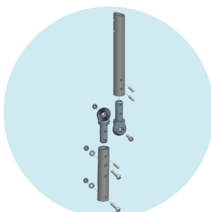
MD10 Rückenlehne winkleinstellbar in 6° Schritten
