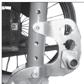
MG86 車軸延長プレート
