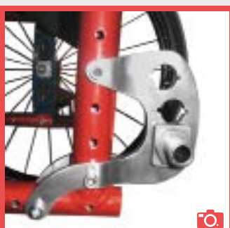
MG 86 Déport de roues arrière
