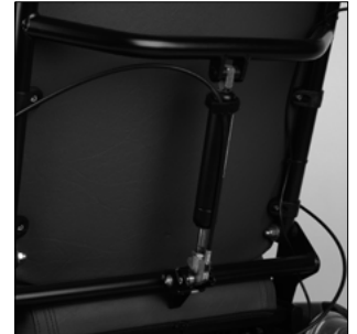
ED 20 Mech. Rücken- winkelverstellung
