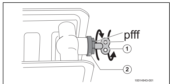
Afb. 9 Ontluchten radiator
