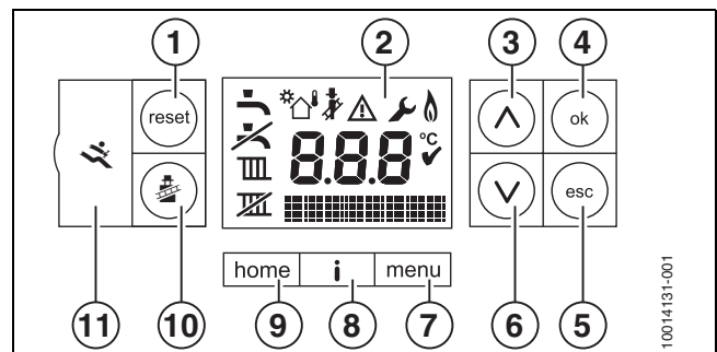
Afb. 5 Bedieningspaneel
