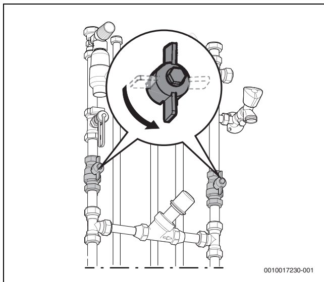
Afb. 4 Serviceafsluiters
