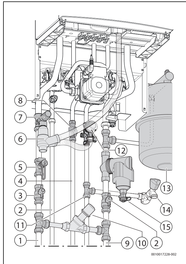
Afb. 2 Overzicht aansluitingen
