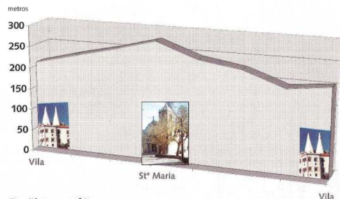
Perfil topográfico
