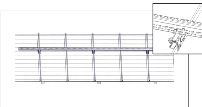
3. För enklare hantering vid panelinfästning: Skenan närmastnock monteras med ryggen upp motnock. Därefter monteras varannan skena med ryggen i motsatt riktning. Det går även att montera samtliga skenor med ryggen motnock.
